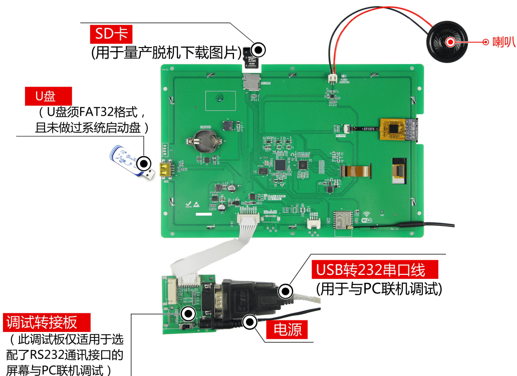
图 1-4 232 调试工具图
