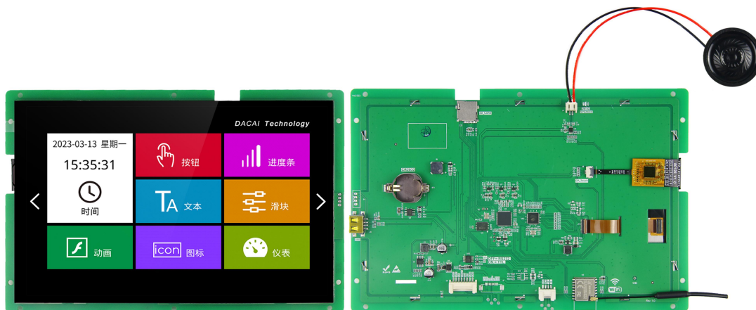
图 1-1 10.1 寸电容触摸参考图
