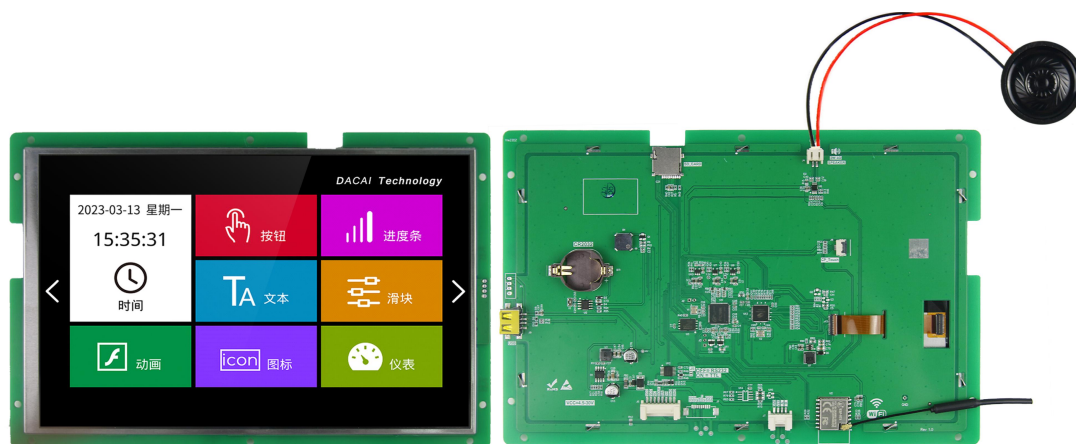
图 1-2 10.1 寸无触摸参考图
