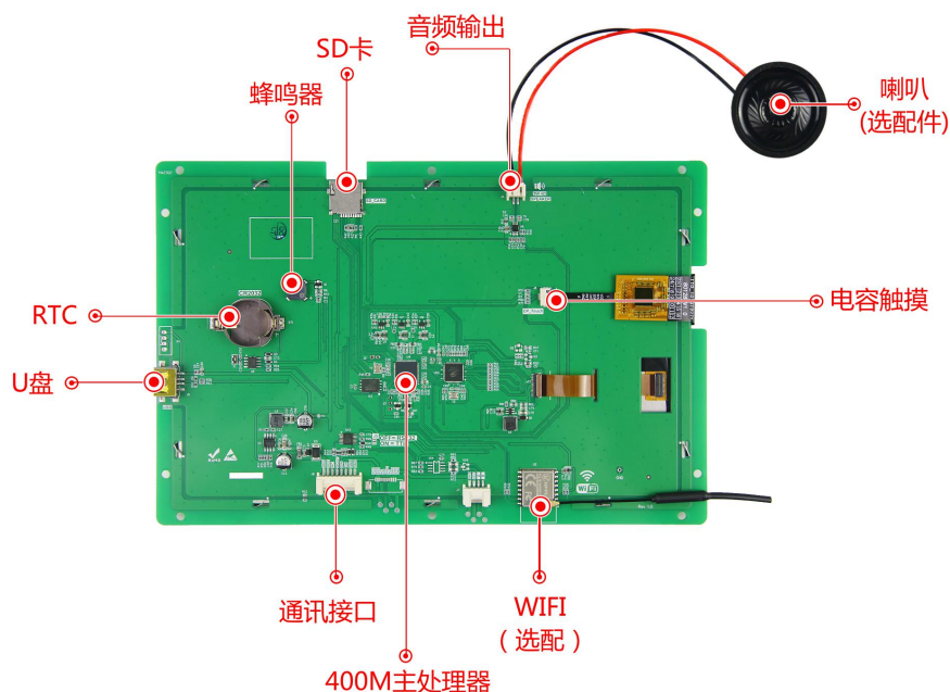
图 1-3 硬件配置图
